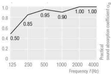
גרף בליעה אקוסטית
