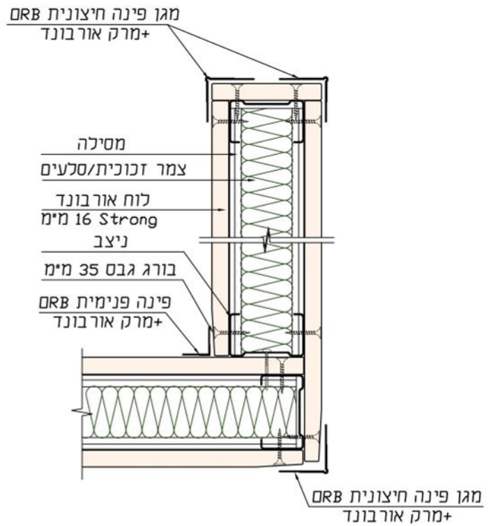
מפגש פינתי וקצה חופשי
