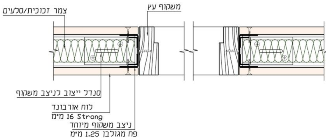
פרט התקנת משקופים לדלתות
