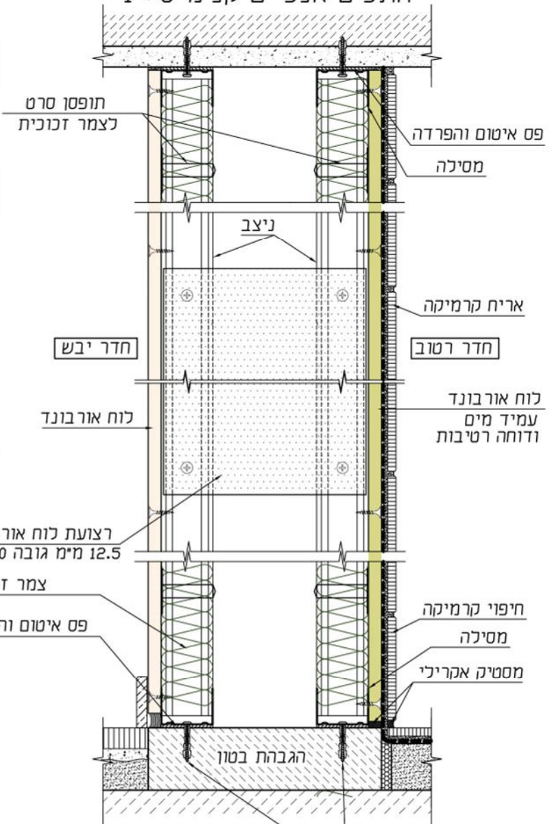
חתכים אנכיים קני"מ 1 : 5
