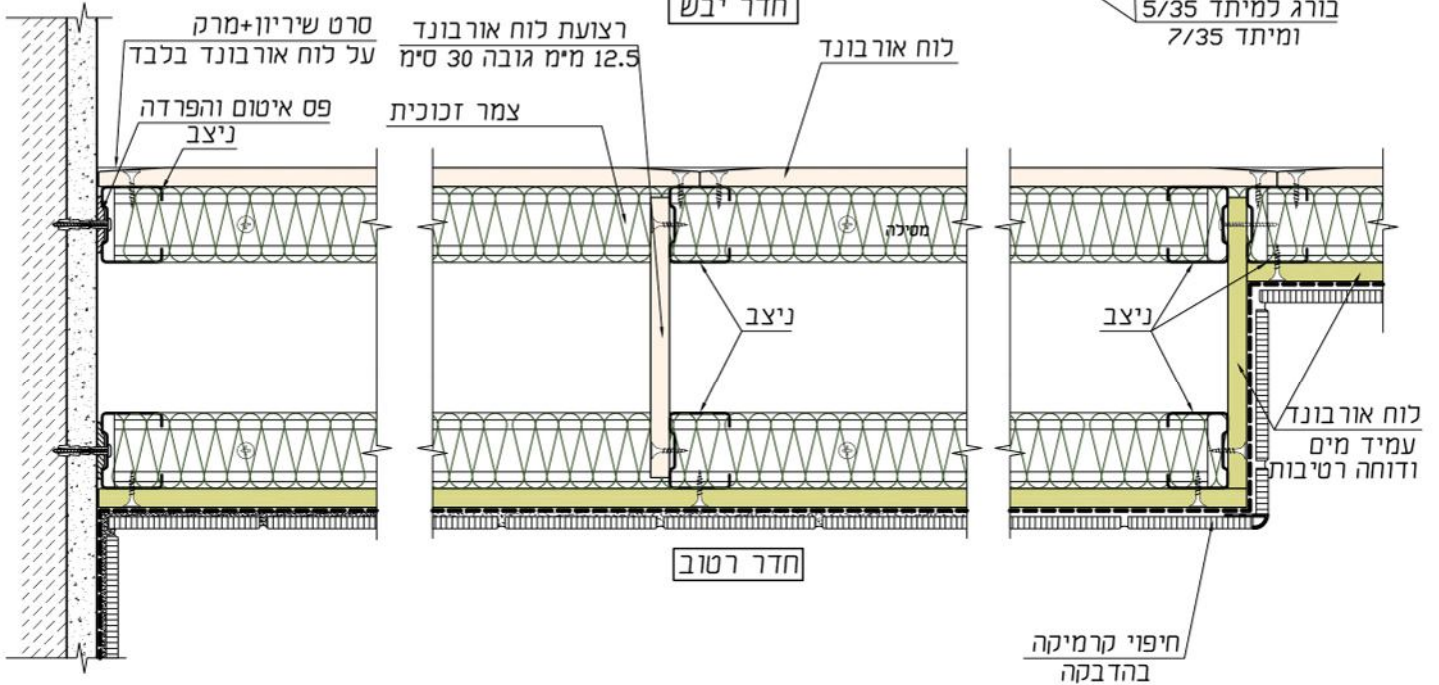
חתכים אופקיים קני"מ 1 : 5
