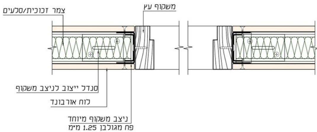
⑦ פרט התקנת משקופים לדלתות
