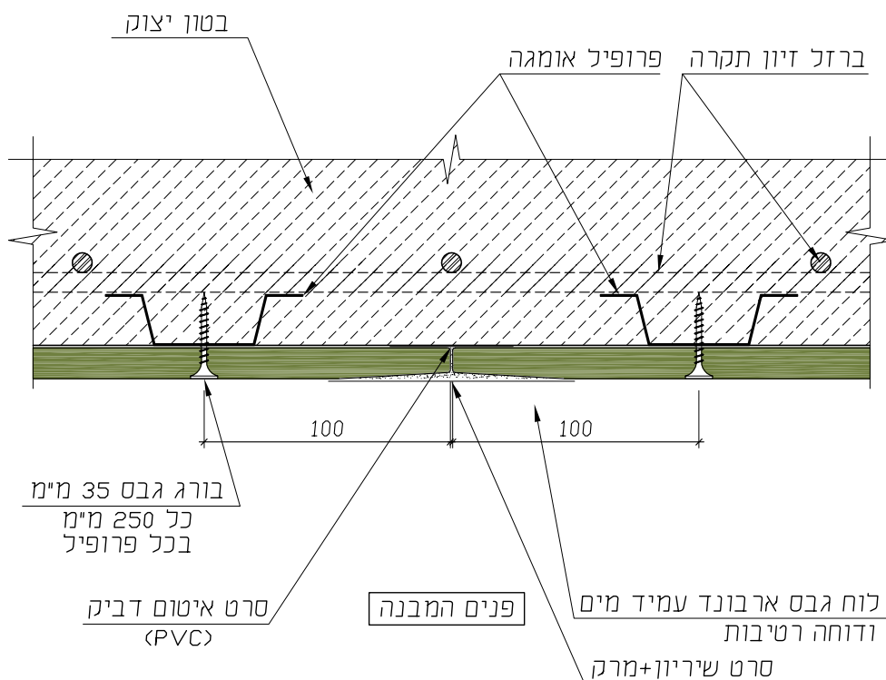
שילוב חיפוי ביציקת שלד הבטון:
